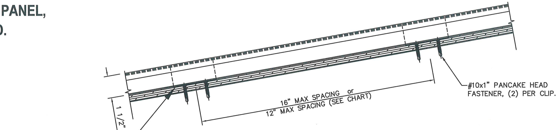
SECTION A-A
